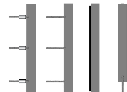
Stud with Spacers Stud Tape Bottom
